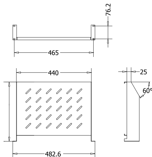
Bandeja 19" negra
