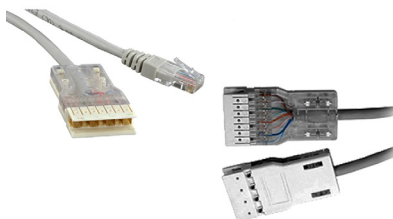
Latiguillo 110/RJ 110/110
