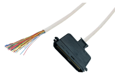
Cables RJ21 Telco 50 M 0°/Libre Laches
