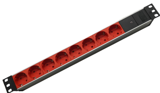
Regleta 19" 1U 8 schukos rojos con piloto LED en aluminio
