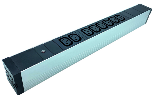
Regleta 19" 1U 8 C13 + 1 C14 con piloto LED en aluminio
